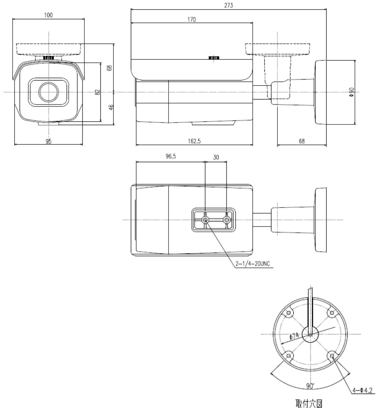
外形寸法図
