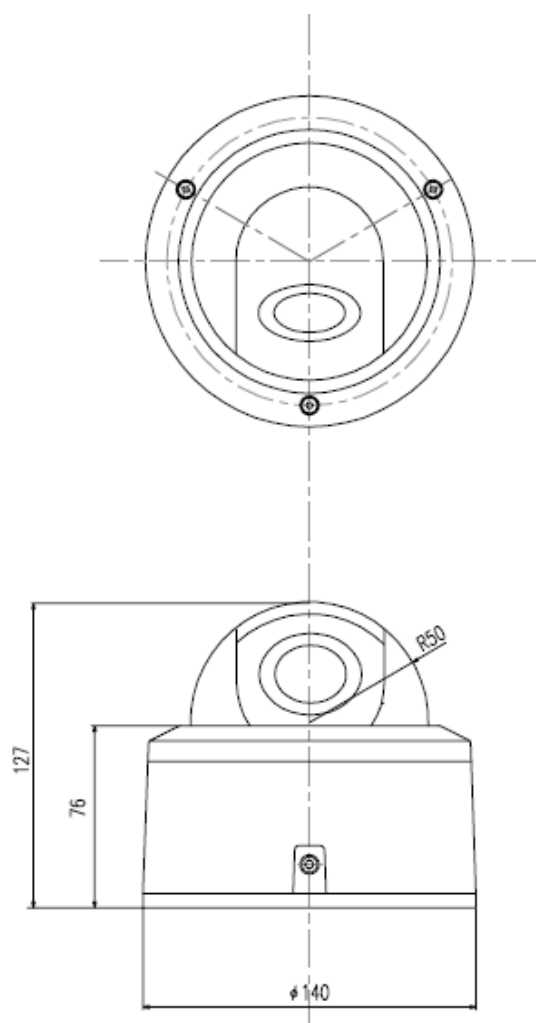
外形寸法図
