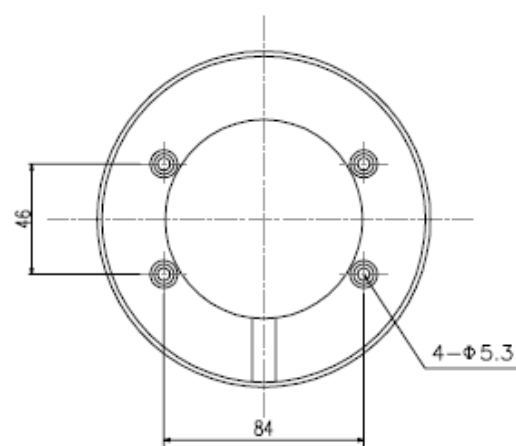
取付穴図
