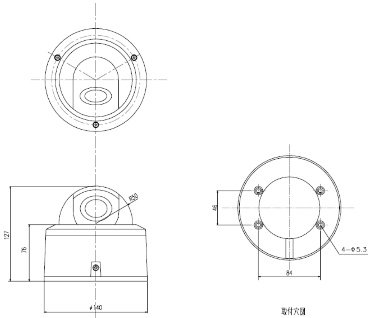
外形寸法図
