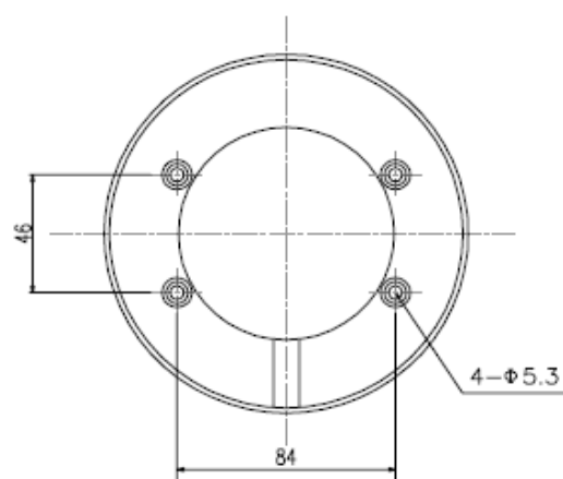
取付穴図
