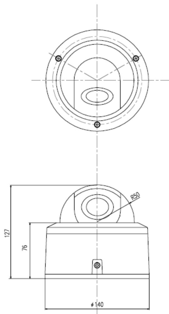
外形寸法図
